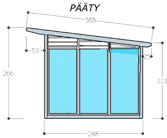
JULKISIVU
